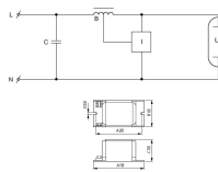
Caractéristiques Philips HID-HeavyDuty BSN 70 L33-TS 230V 50Hz HD1-118
