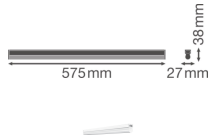
Caract ristiques Ledvance R glette LED Linear Compact 10W 1000lm - 840 Blanc Froid | 60cm
