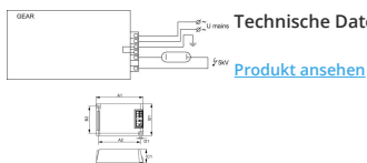
Technische Daten Philips HID-PV C 35 /S CDM 220-240V 50/60Hz für 35W
